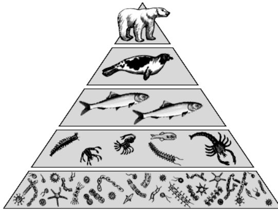
Рисунок 1.2. – Приклад трофічного ланцюга
