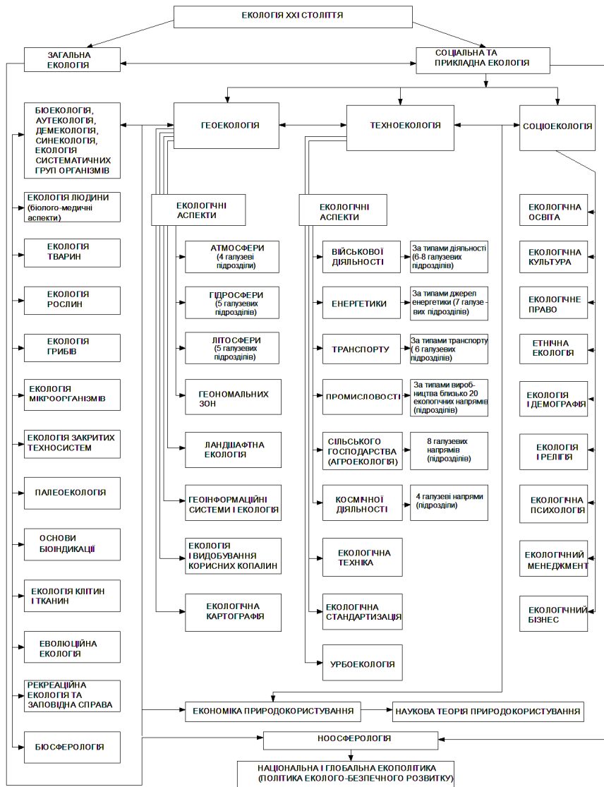
Рисунок 1.1. – Схема структуризації сучасної екології
