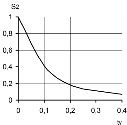
Рисунок 2.5. – Безрозмірний коефіцієнт S_2 , що враховує зменшення приземної концентрації на відстані ( y ) від вітрової осі на лінії, перпендикулярної до цієї осі
