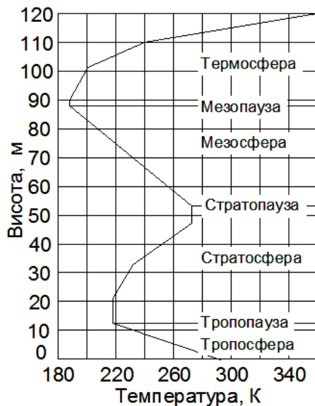
Рисунок – 2.2. Структура атмосфери
