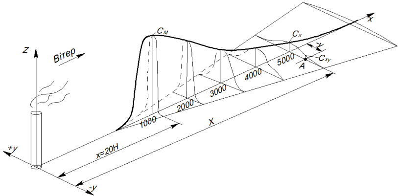
Рисунок 2.3. – Аксонетрична схема приземної концентрації та точкового джерела забруднення
