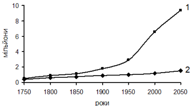
1 – країни, що розвиваються; 2 – розвинені країни Рисунок 4.2. – Середньорічний приріст населення земної кулі
